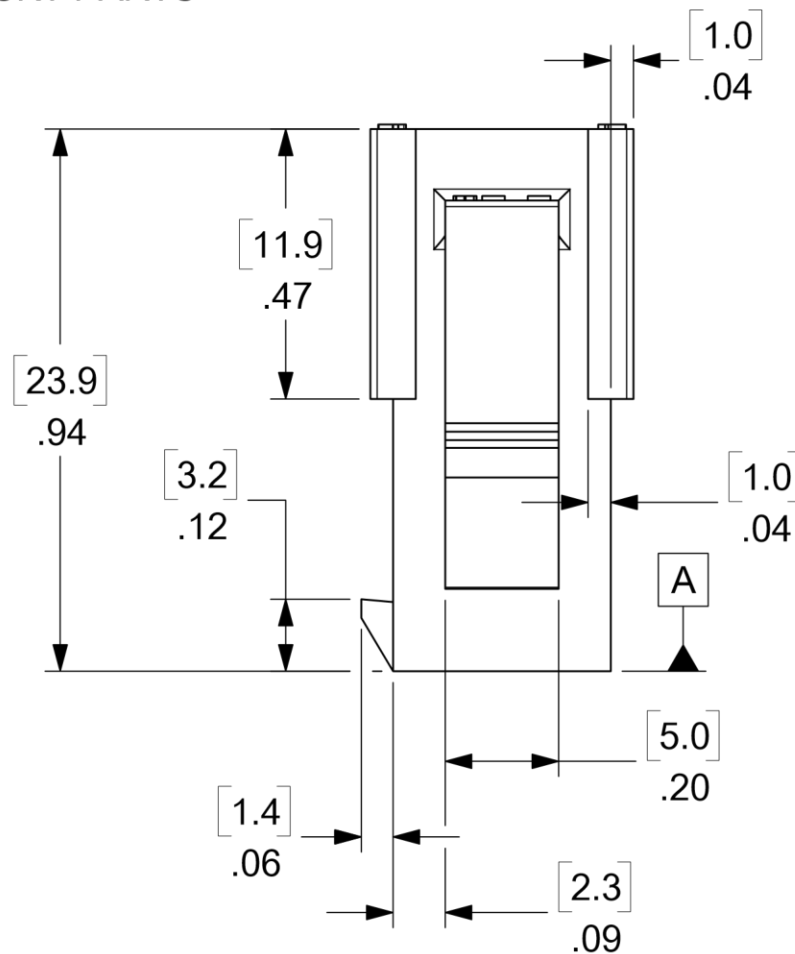
8 CKT SHOWN
