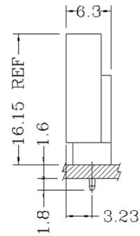
S-Type/直插型
